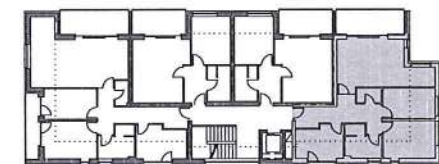
OBBERGESCHOSS 2 SECONDO PIANO
